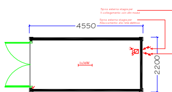
CONTAINER 15' F.S.
